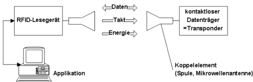
Funktionsweise Transpondersystem
